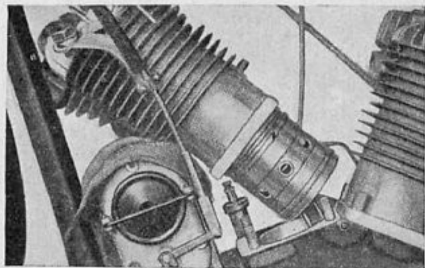
Удаление цилиндров на моторах без с'емной головки
